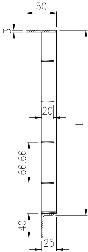
Section A-A
