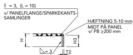
SNIT C-C KANTSTÅL PÅ TVÆRS AF PANEL OG I UDSKÆRINGER
