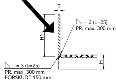
SNIT B-B SPARKEKANT PÅ LANGS AF PANEL
