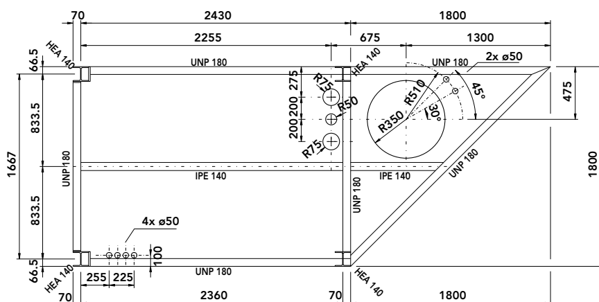
PLAN AF UNDERKONSTRUKTION
