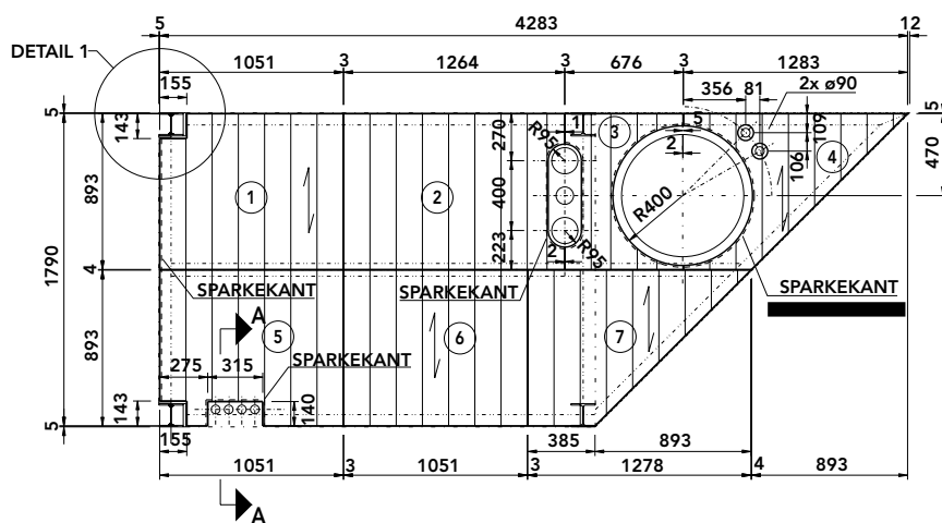
PLAN AF RISTEDÆK
