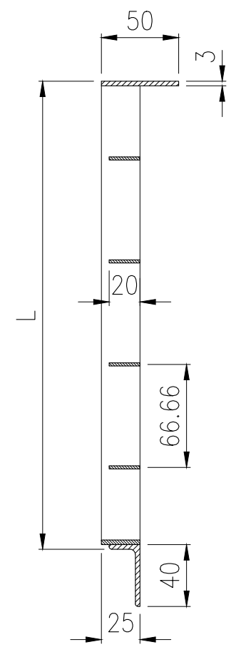
Section A-A
