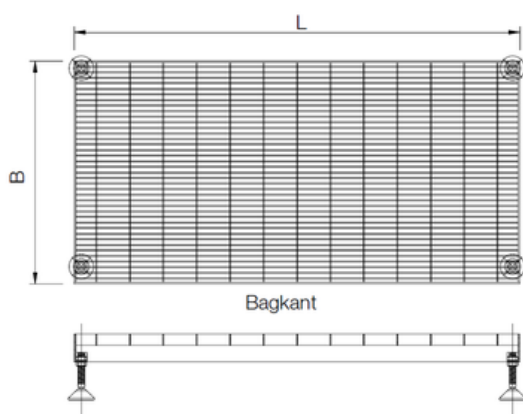
Trinrist Futura
