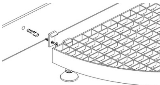
Beslag til fastgørelse i mur
