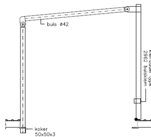
Zijaanzicht open
